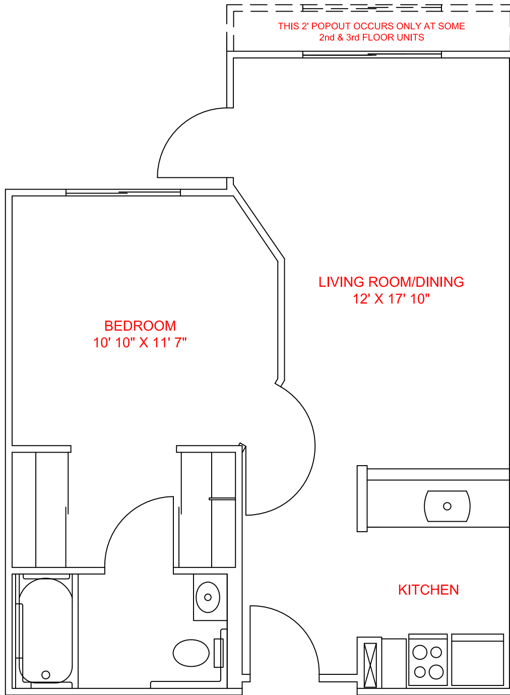
TYPE B - 1 BEDROOM
